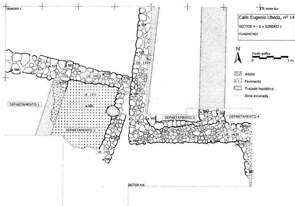
Figura 2. Planta con los restos de dos edificios del segundo cuarto del siglo II a.C., hallados en las excavaciones arqueológicas de la calle Eugenio Úbeda, 12-14, Lorca.
